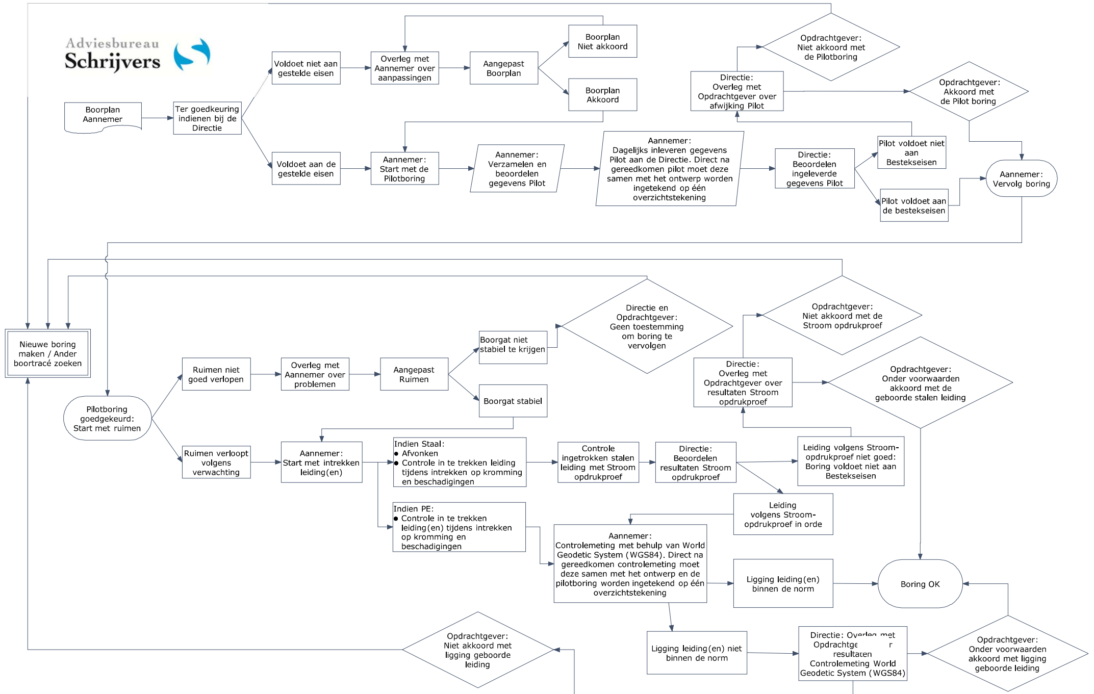
Horizontaal gestuurde boring: Pilot- Ruimer- en intrekfase
